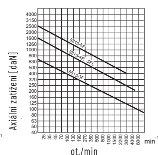
Axiální zatížení Životnost ložisek - 2000h
