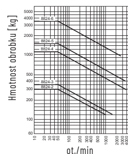
Radiální zatížení Životnost ložisek - 2000h
