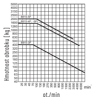
Radiální zatížení Životnost ložisek - 2000h
