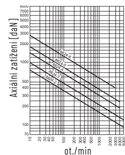
Axiální zatížení Životnost ložisek - 2000h
