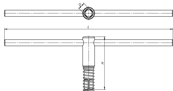
Pro typ • 3105, 32**, 35**, 36**, 37**, 38**, 43**
