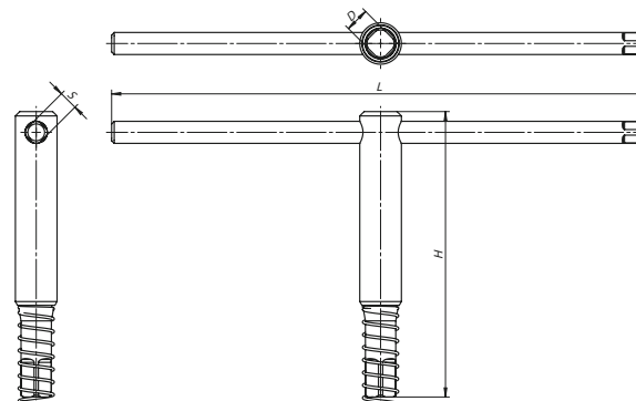
Pro typ • 45**, 46**, 47**, 48**
